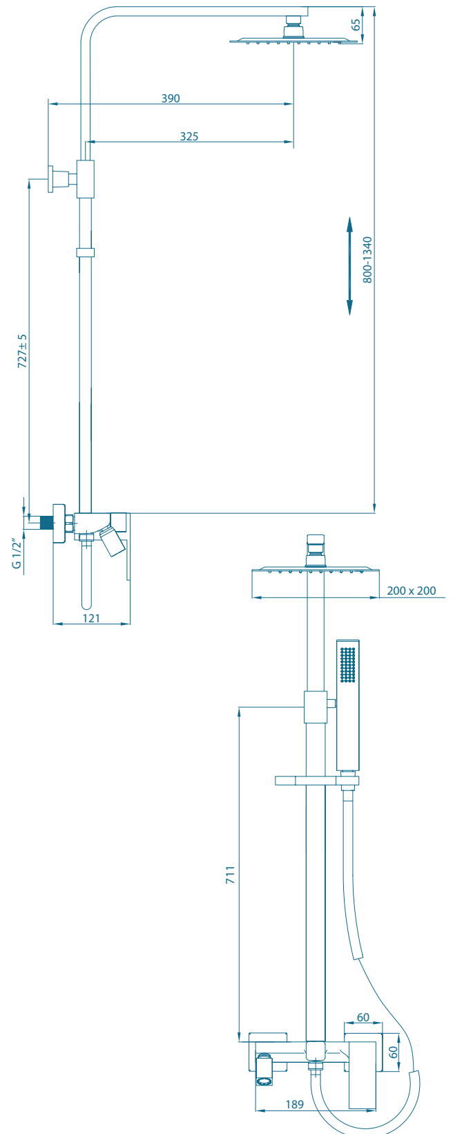
Desenho técnico (mm)
