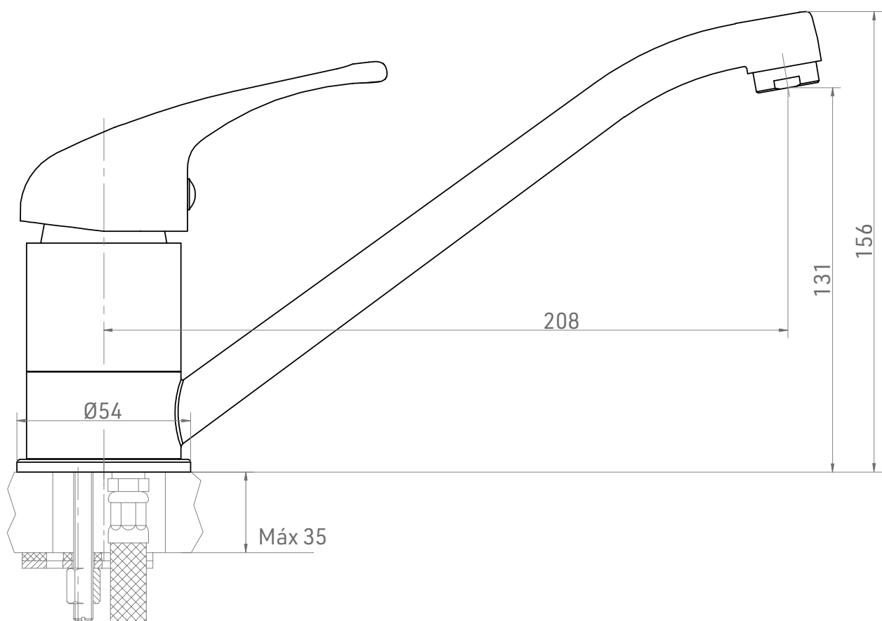
Desenho técnico
