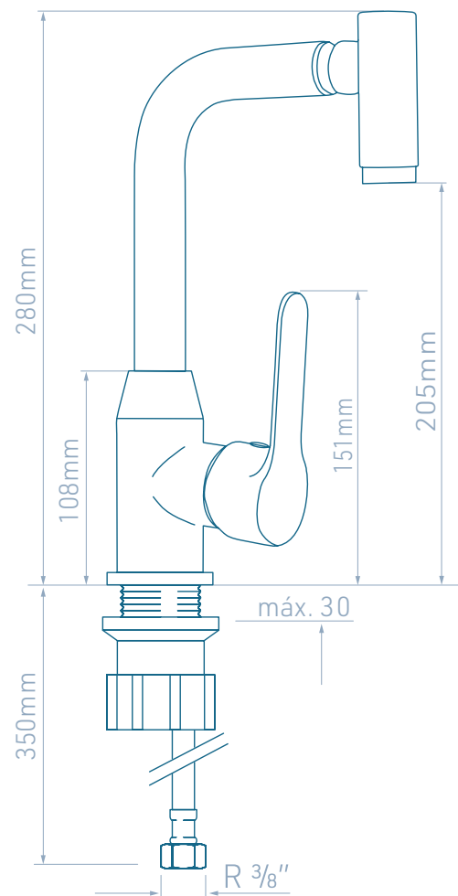
Desenho técnico (mm)
