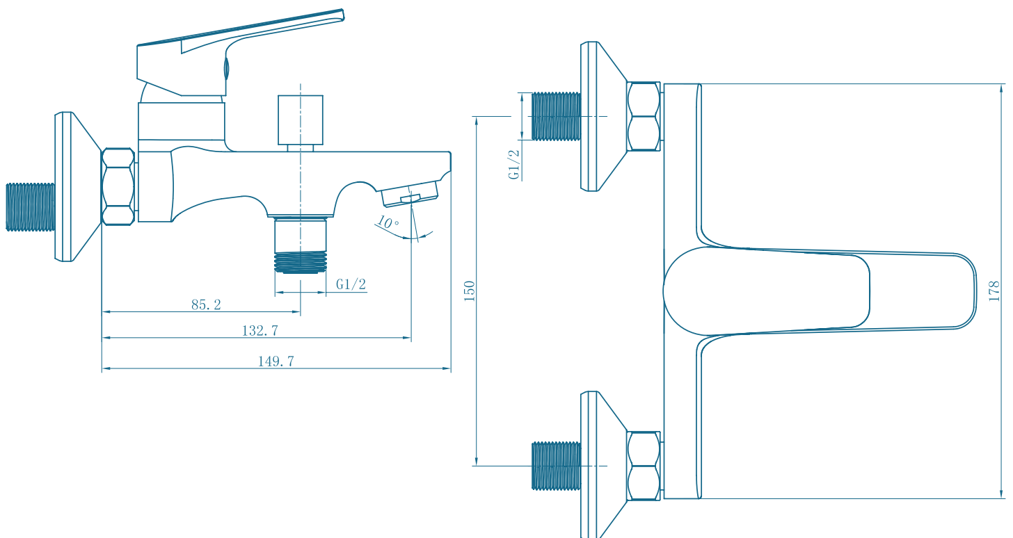
Desenho técnico
